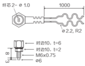
EFG-QD31QP-n(多合一反射光纤n=4、6、8、10)
