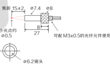
EFG-4HA (15mm处小光斑)
