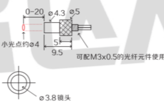
EFG-3HA (平行光斑)
