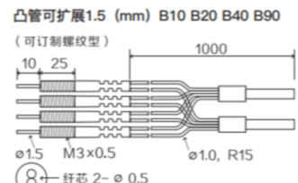
EFG-QD31QP-n(多合一反射光纤n=4、6、8、10)
